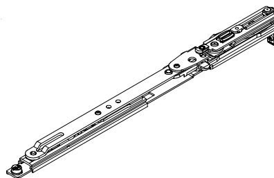
DK-Schere DK stay 3.1 – 300, 60 kg 3.2 – 400, 130 kg 3.14 – 400, 160 kg
